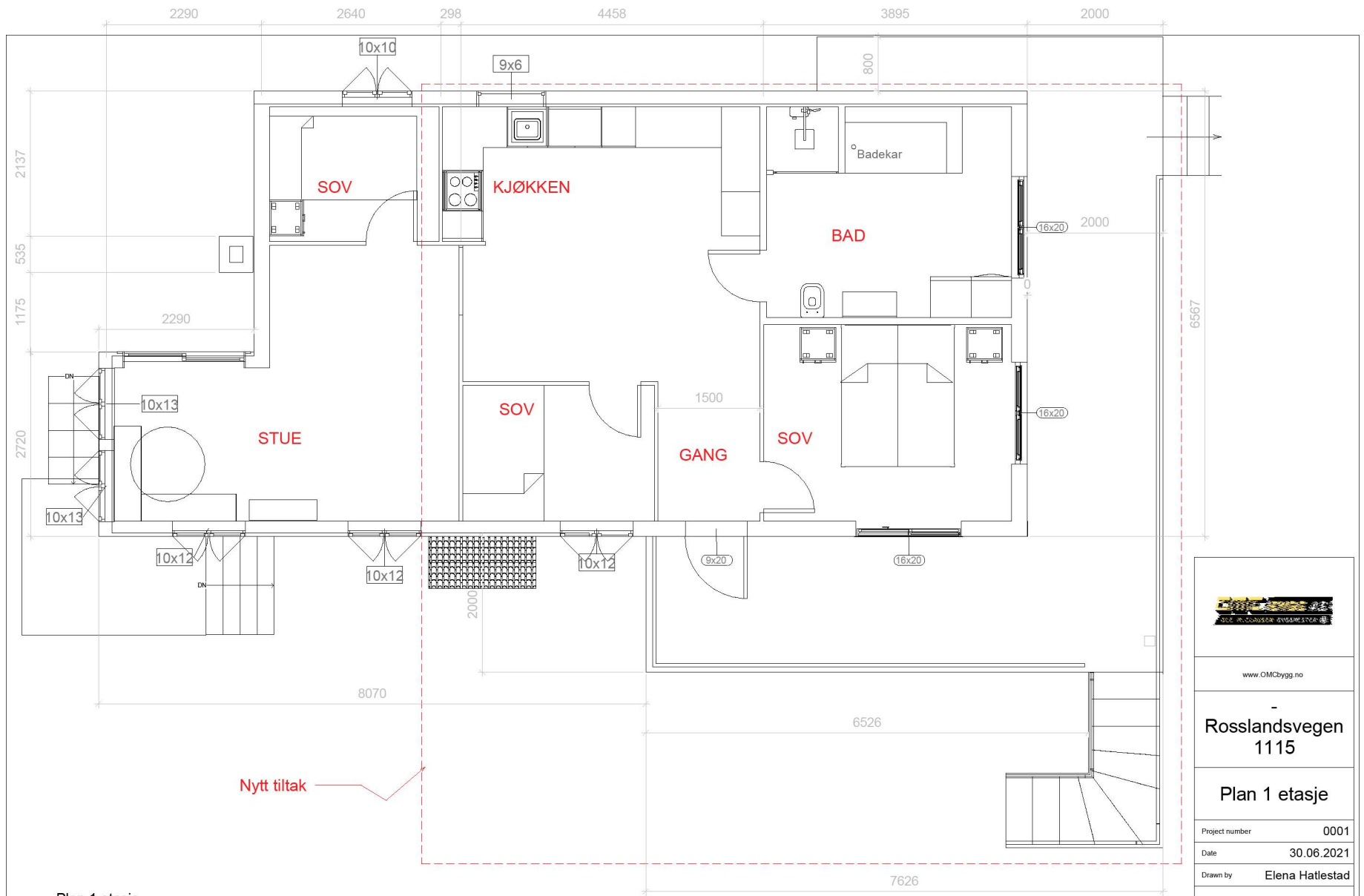
1 Plan 1 etasje 1 : 25
