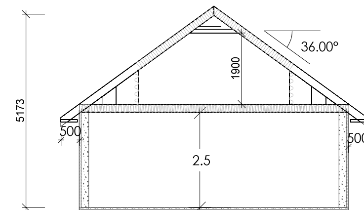
Snitt A-A
