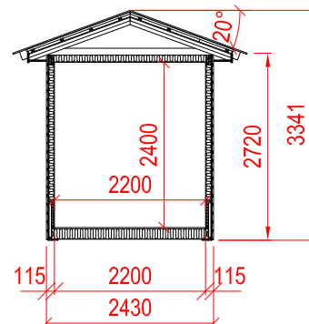
Snitt A-A
