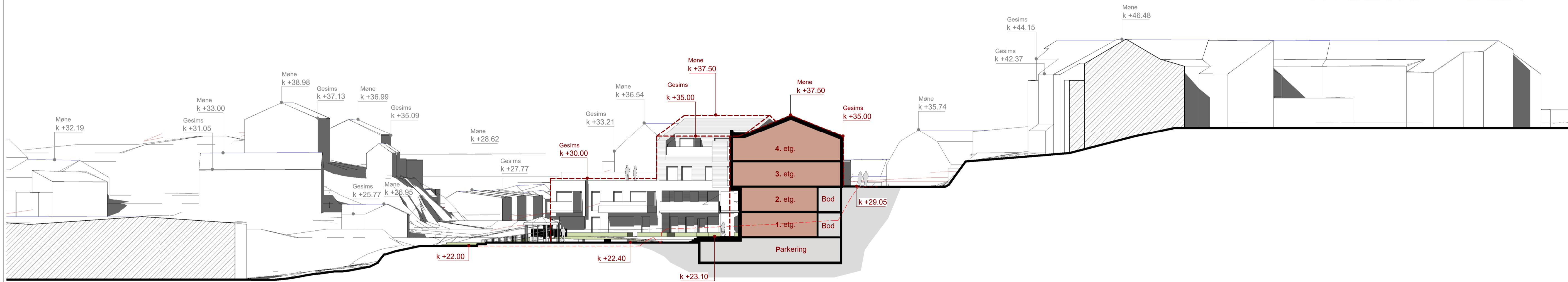
Snitt 3-3 1 : 250
