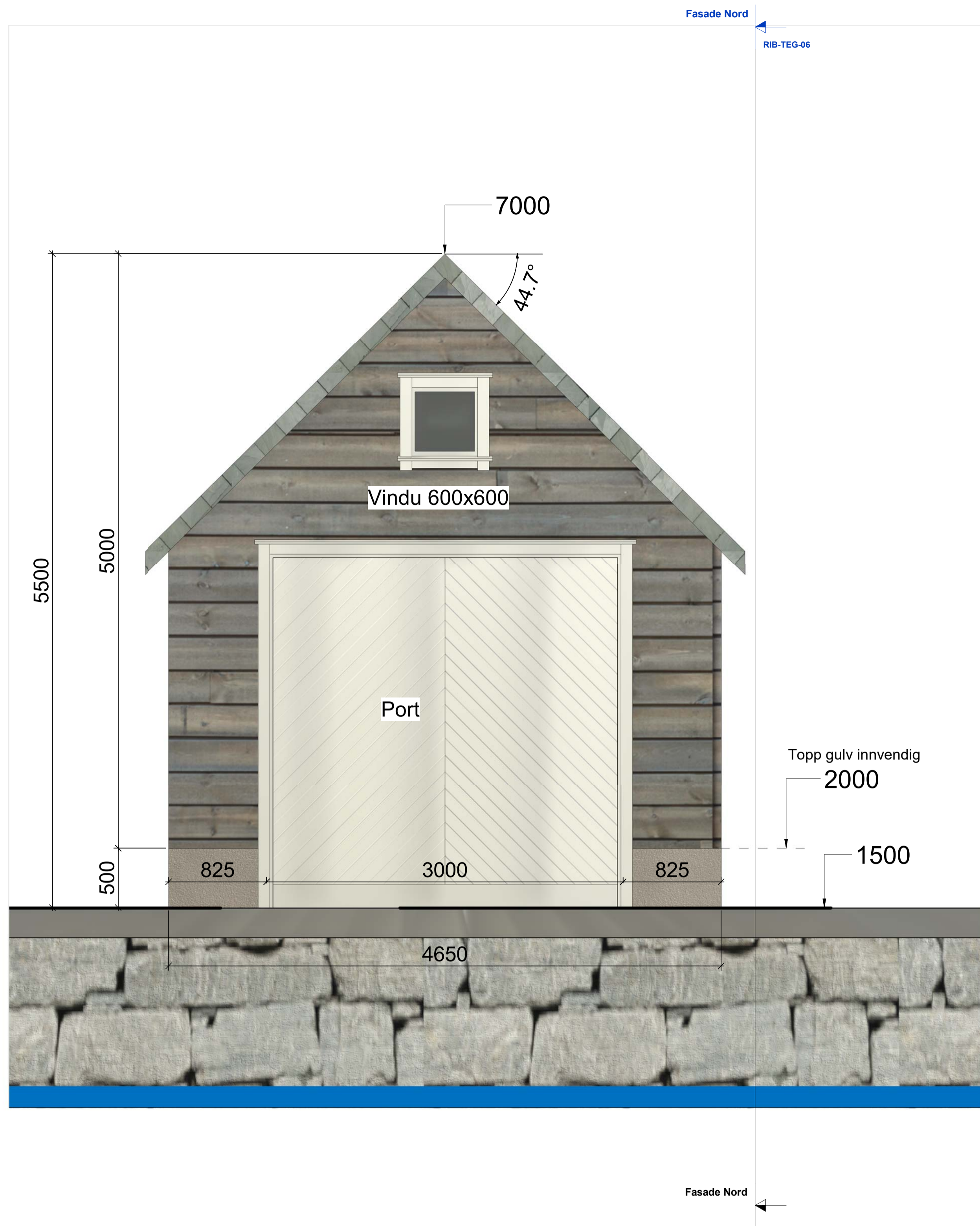
Oppriss Front/Fasade øst 1:25
