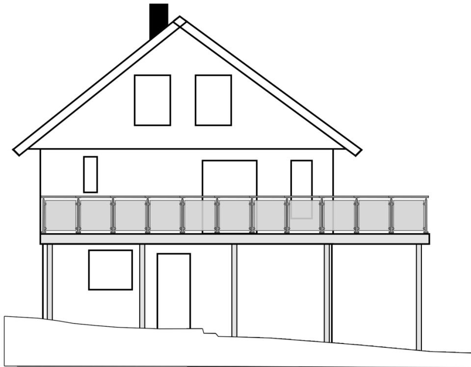
Fasade NORD-VEST 1:100
