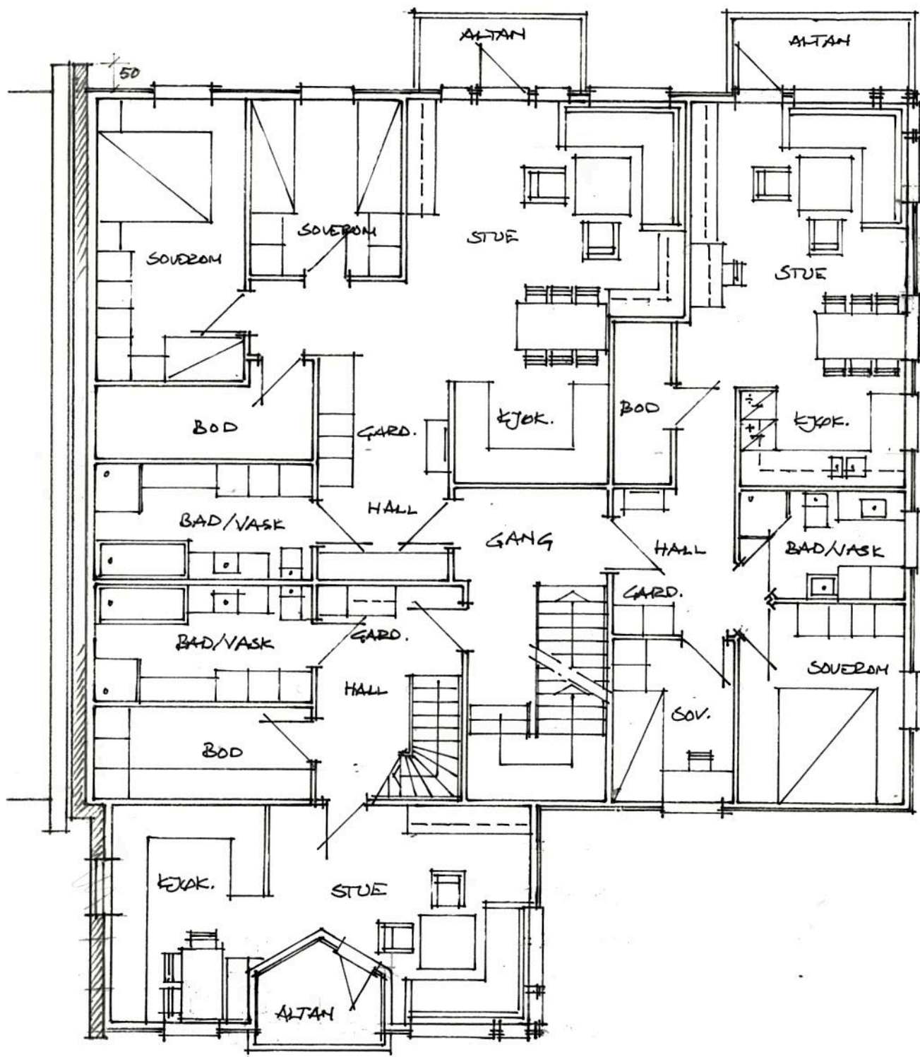
PLAN 2 ETG. M 1:100
