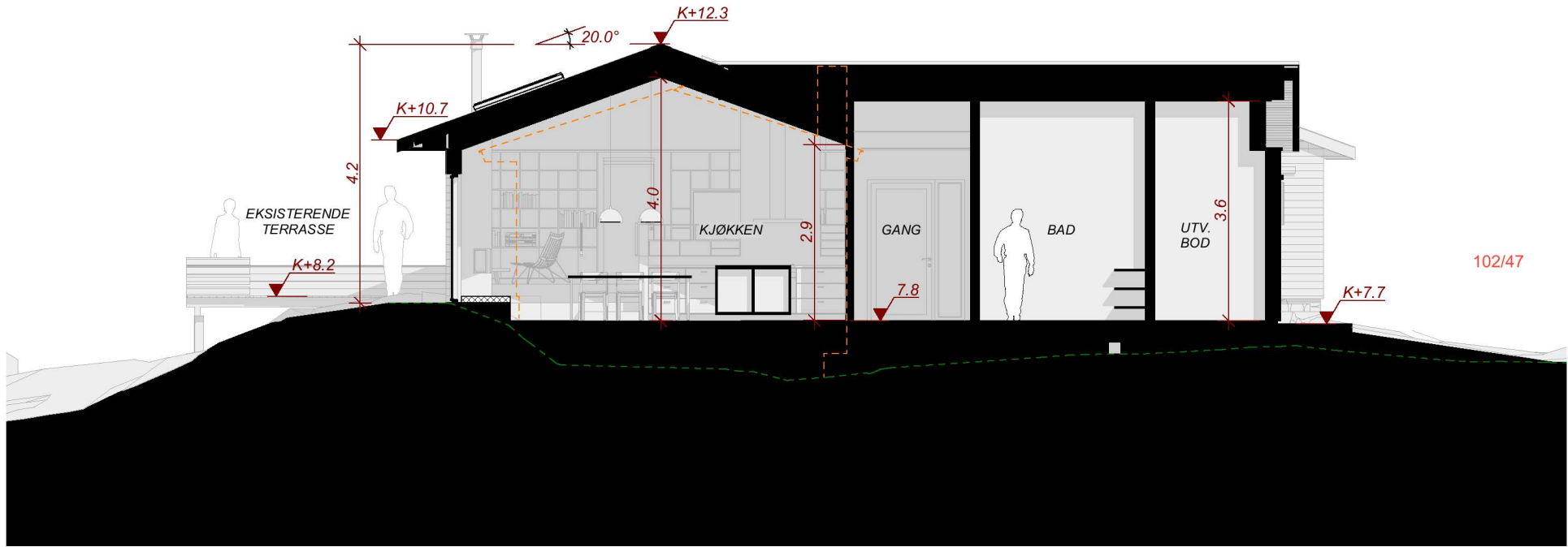
Snitt C - Planlagt
