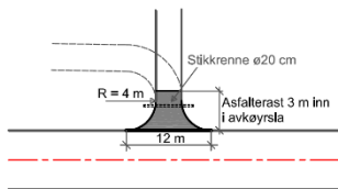
Detaljteikning for avkjørsle
