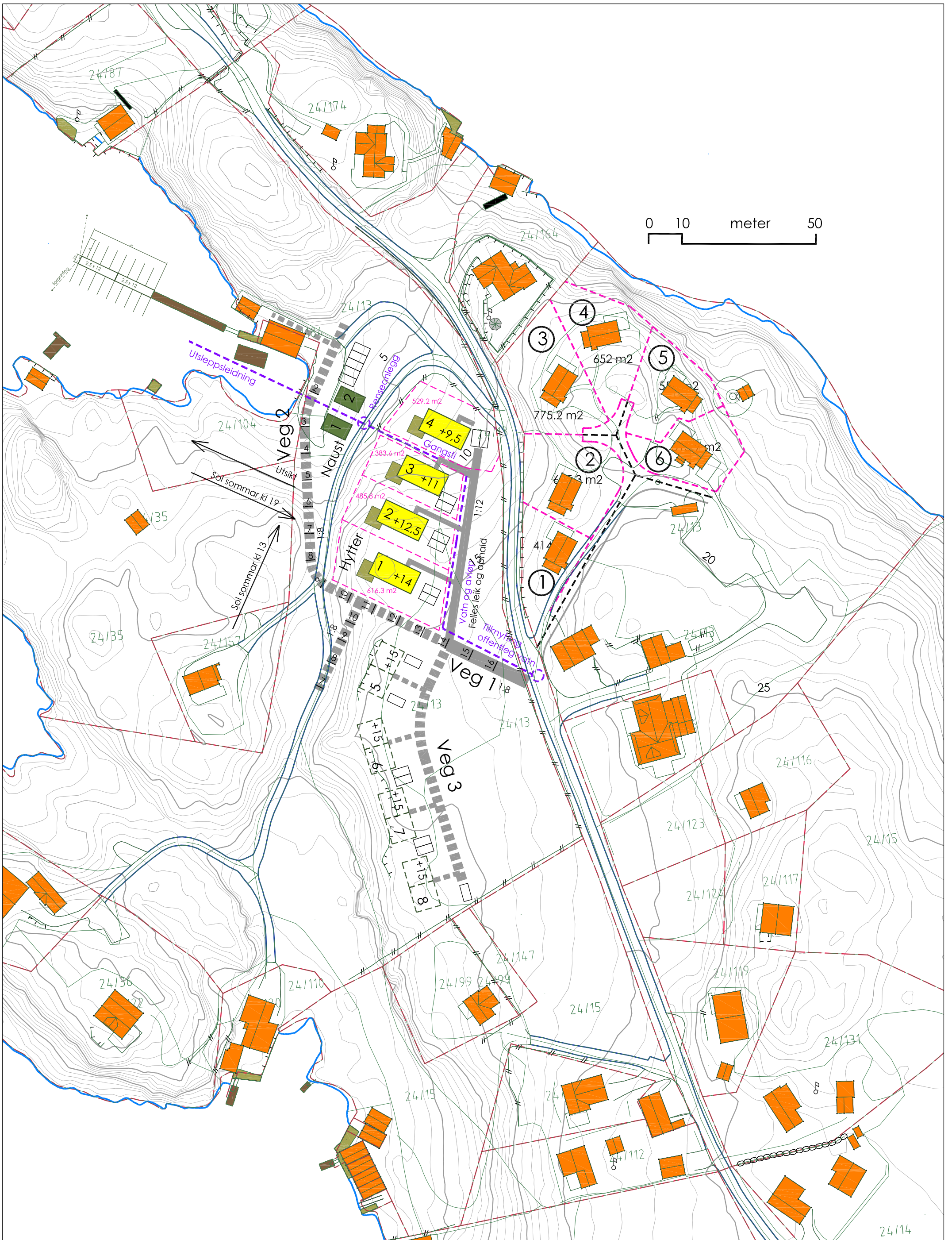
Gbnr. 424/13 Nordbø Hyttetun 2 naust og 4 utleiebustader. Samla situasjonsplan 12. oktober 2021 / Vidar Mjøs
