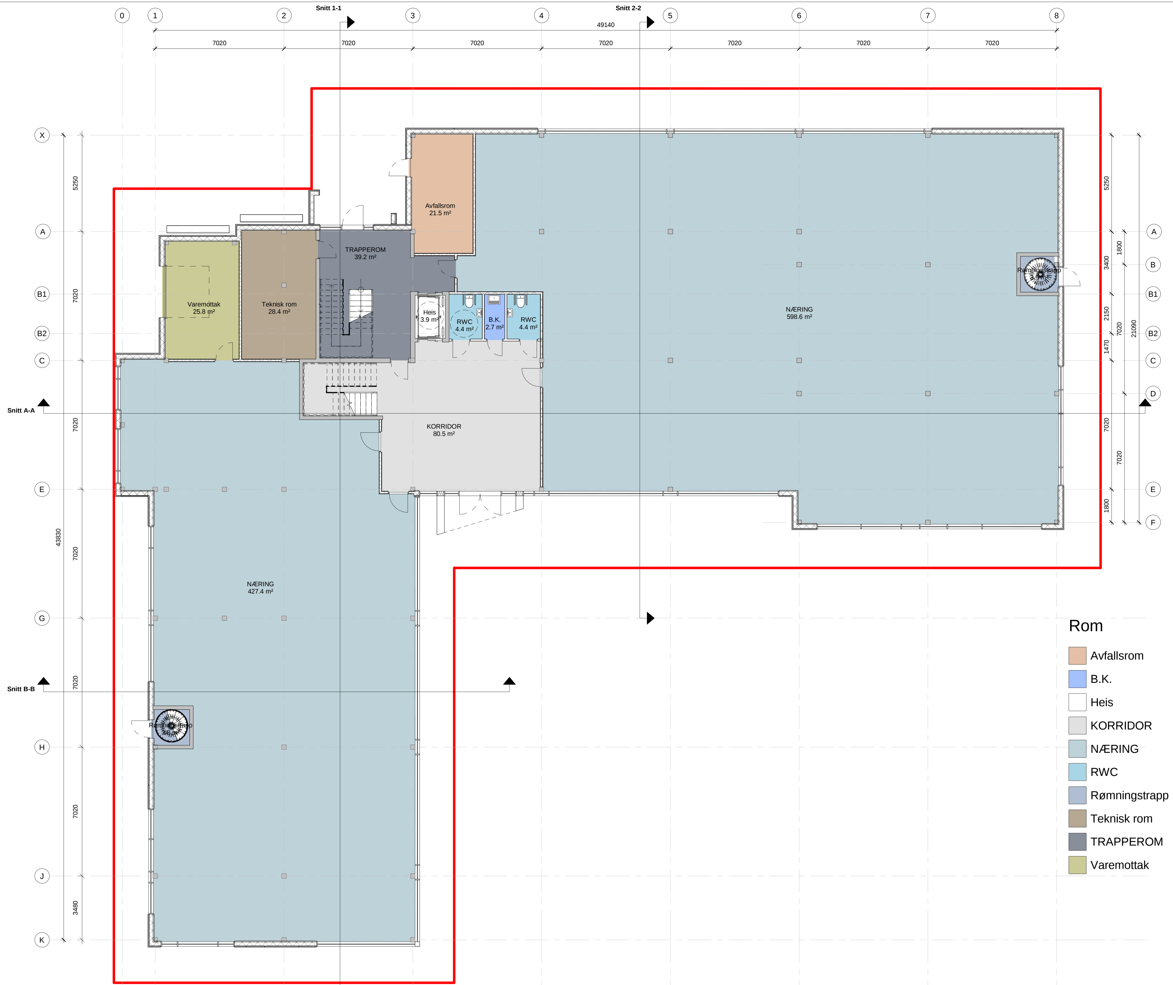
1 Plan 01 1 : 100
