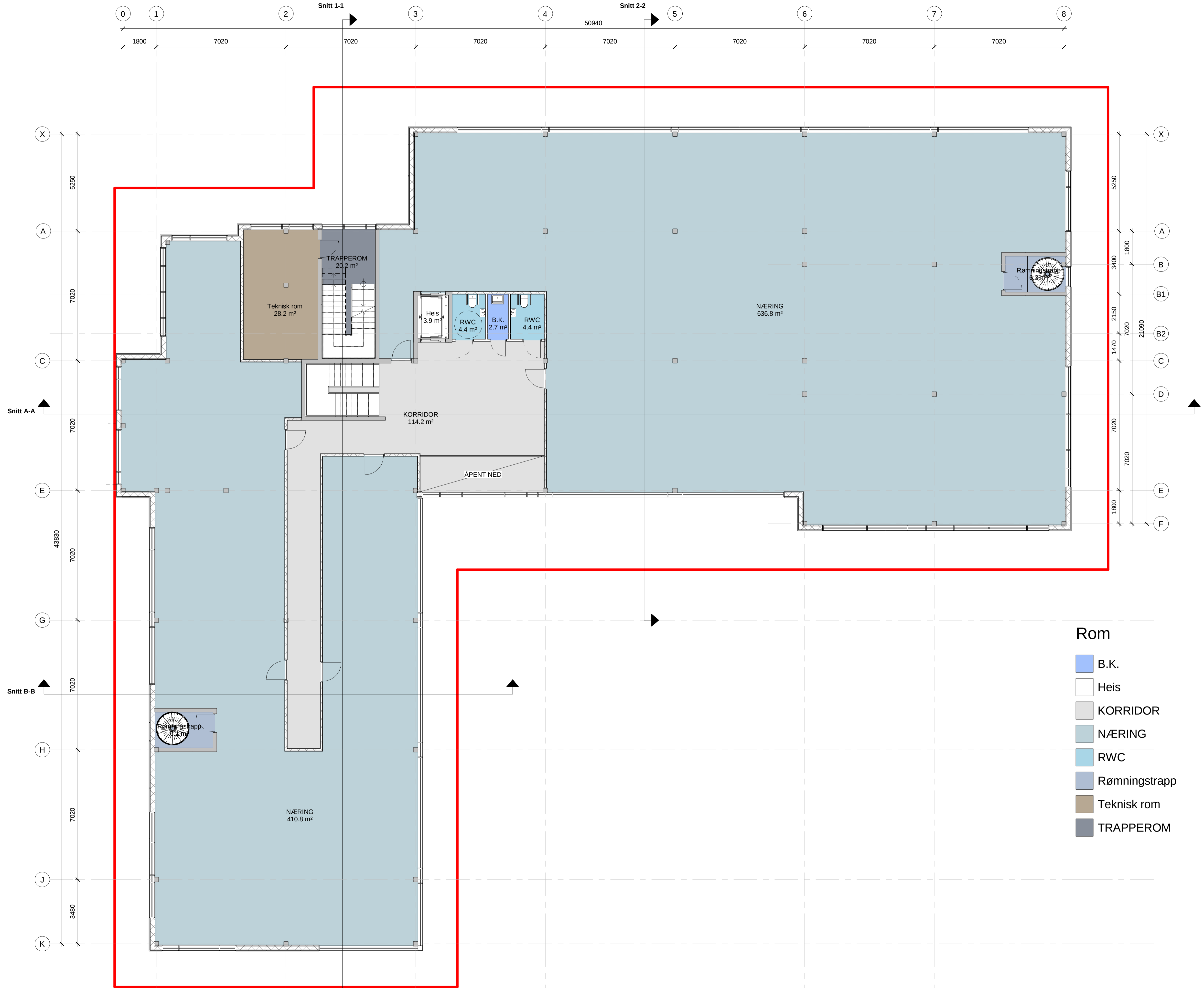
1 Plan 02 1 : 100
