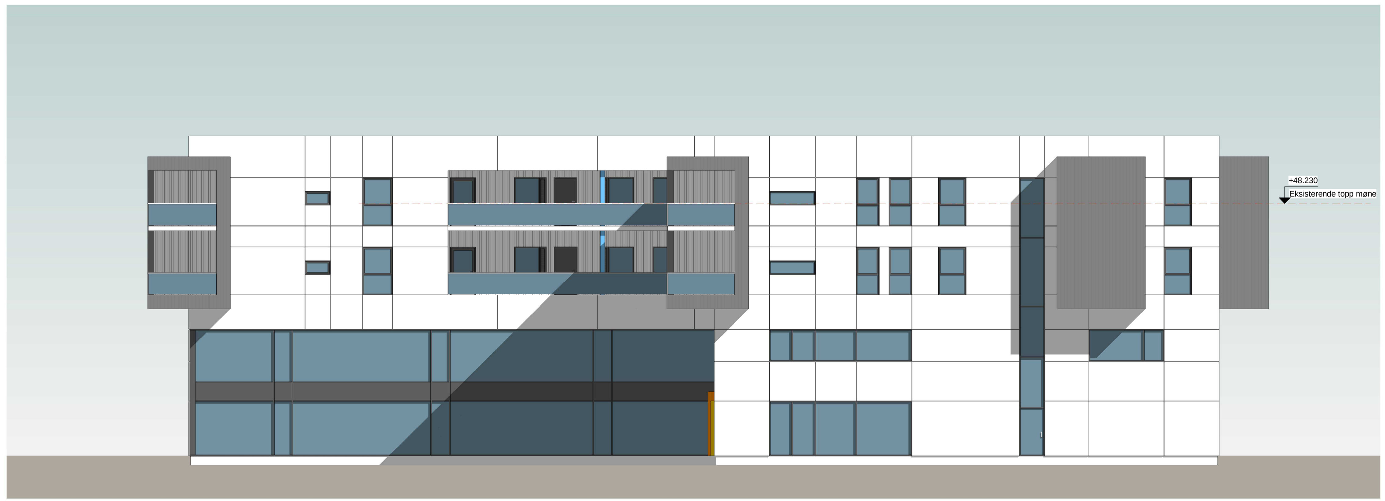
2 Nordøst 1 : 100
