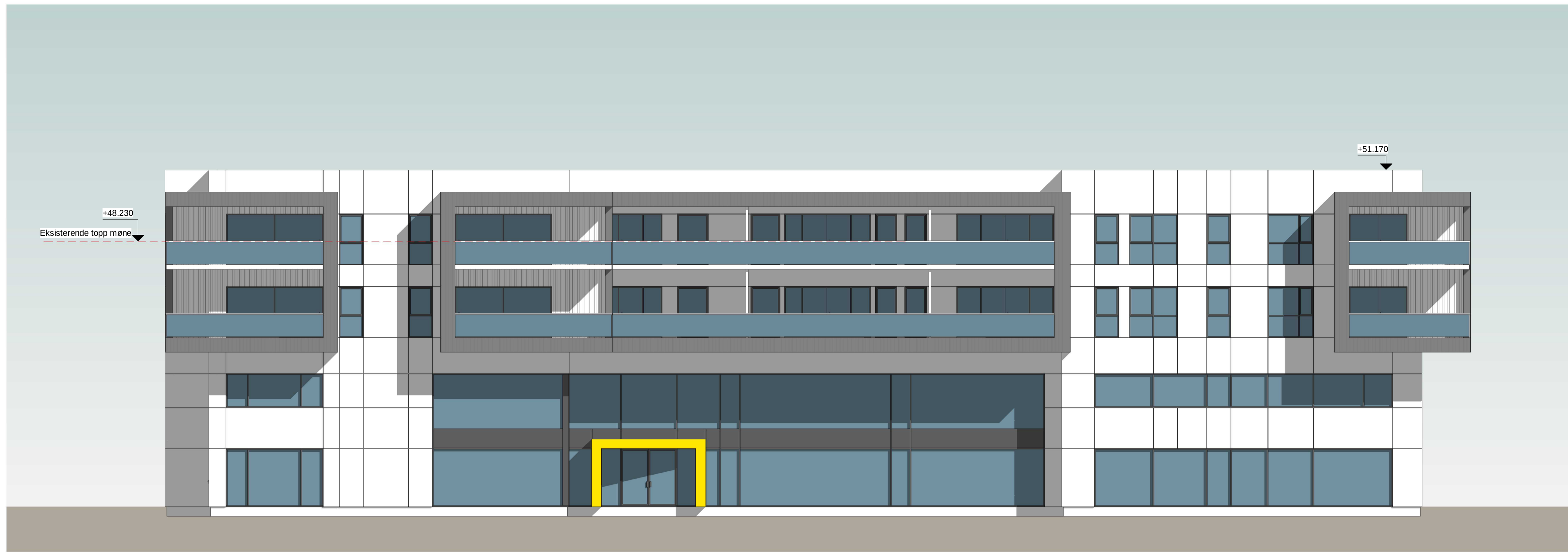
1 Sørøst 1 : 100
