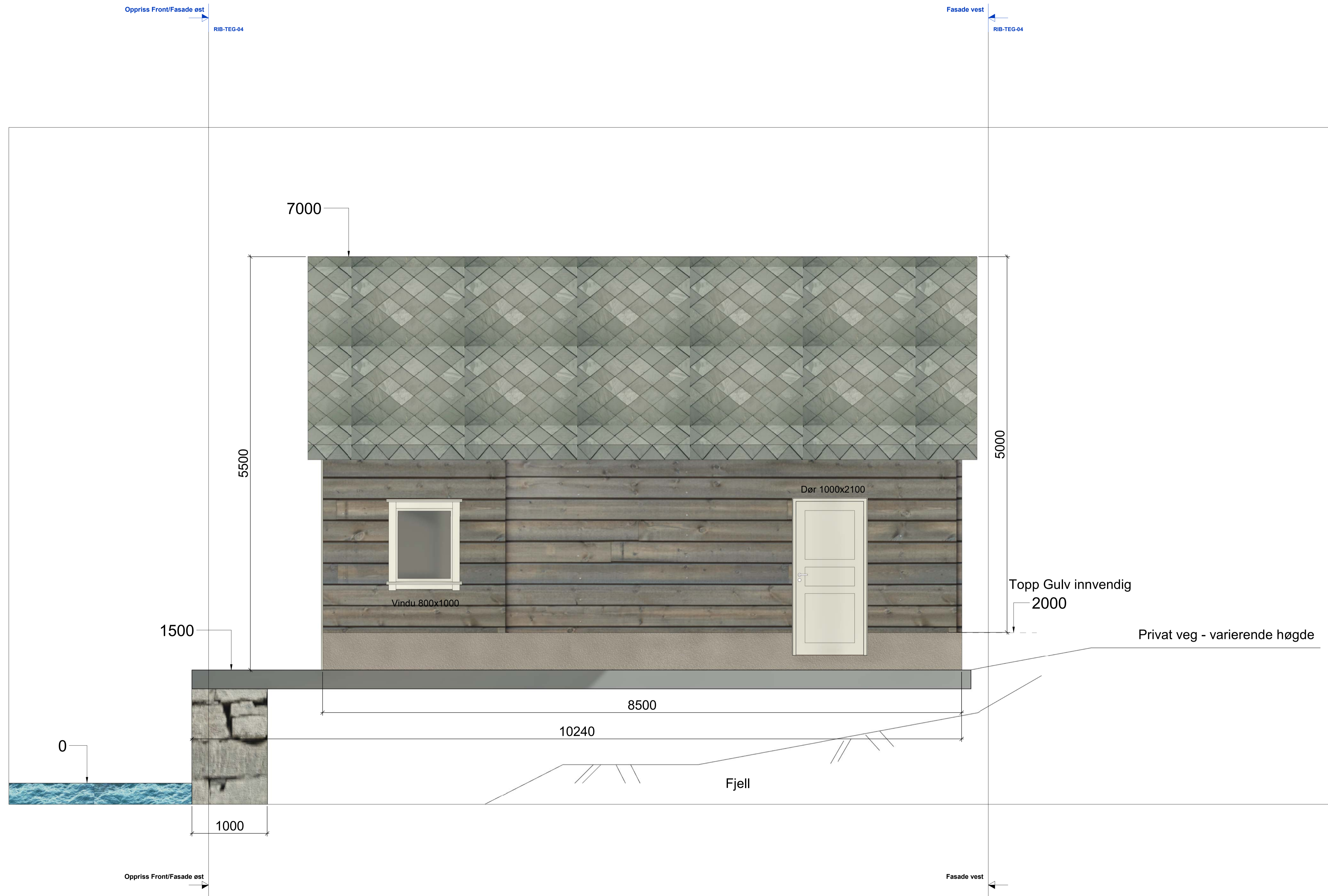
Fasade Nord 1 : 25
