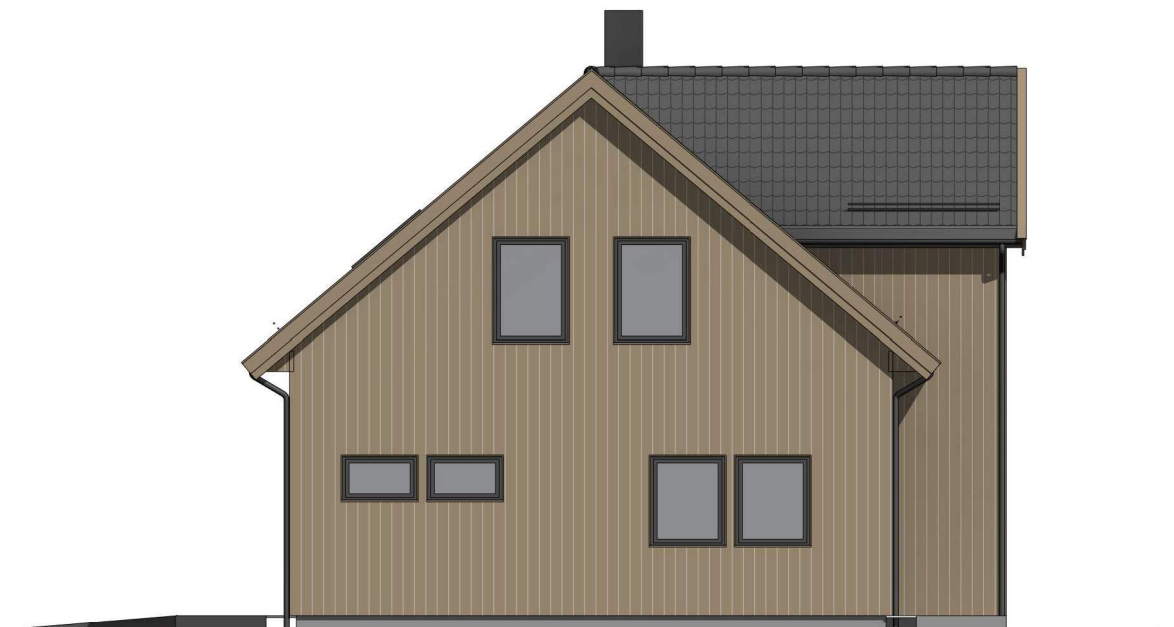
ssø 1 : 100
