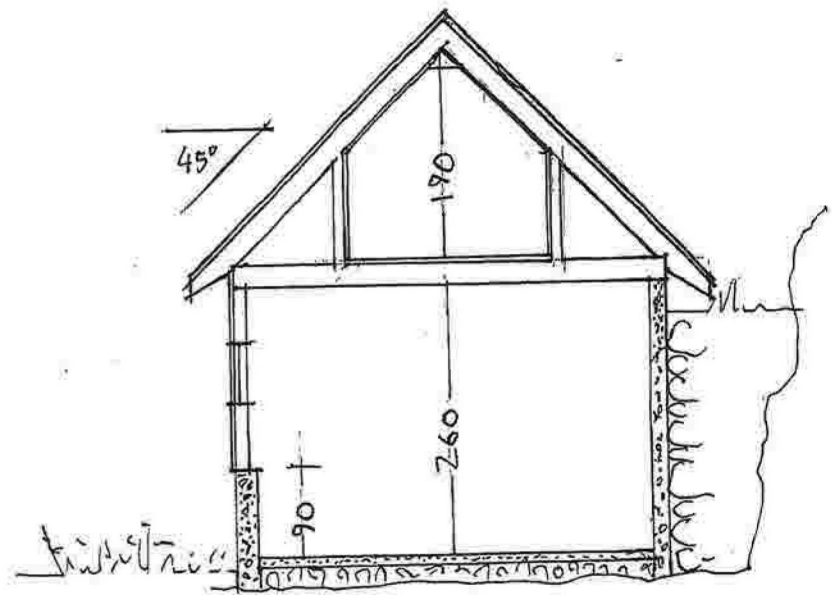
SNITT
