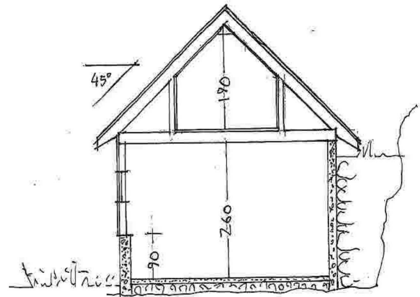
SNITT
