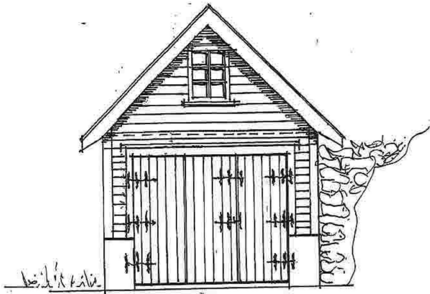
FASADE MOT SYD
