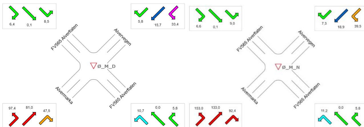
Figur 3-18 Metningsgrad - Østre kryss morgen – Dagens (venstre) og fremtidig situasjon (høyre)
