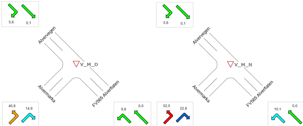
Figur 3-13 Forsinkelse - Vestre kryss morgen – Dagens (venstre) og fremtidig situasjon (høyre)
