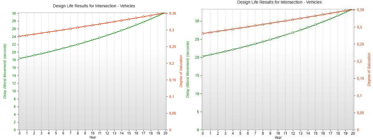
Figur 3-17 Vestre kryss: Fremskrivning av trafikkvolum – Resultater for forsinkelse og metningsgrad i ettermiddagsrush. Uten (venstre) og med (høyre) utvidelse av skolen.
