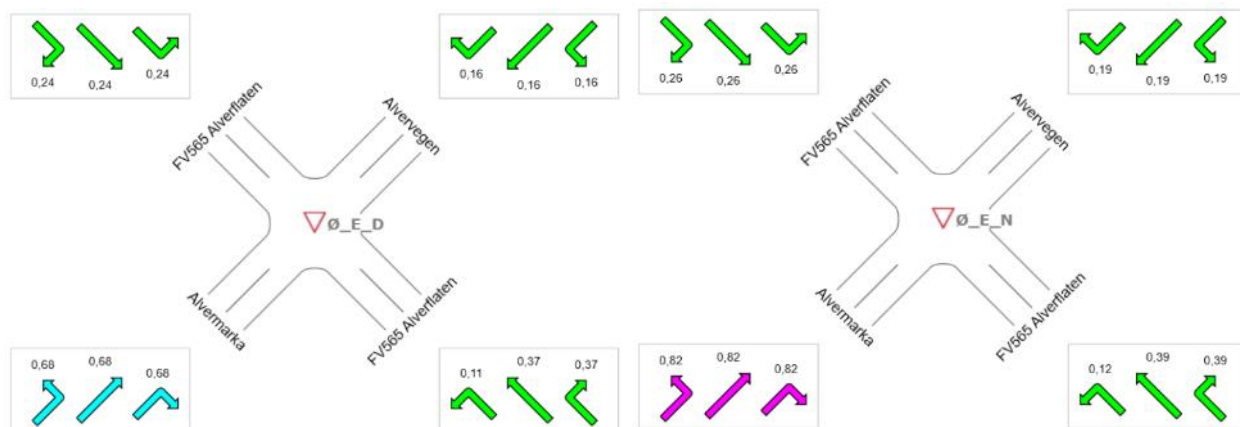
Figur 3-21 Metningsgrad - Østre kryss ettermiddag – Dagens (venstre) og fremtidig situasjon (høyre)
