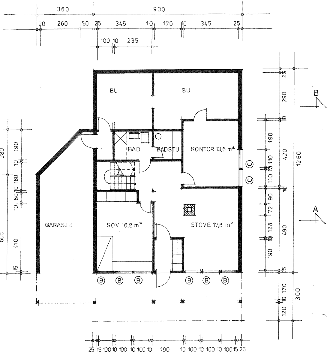
PLAN AV KJELLAR
