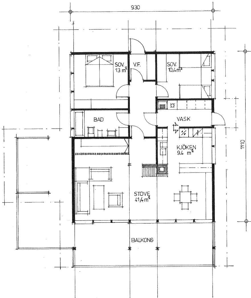
PLAN AV 1. HÖGDA
