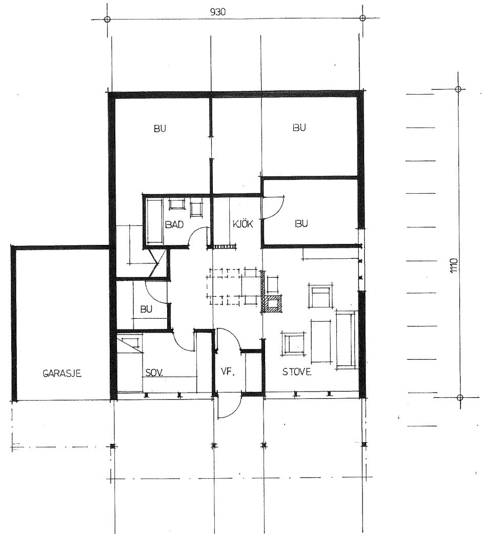
PLAN AV KJELLAR
