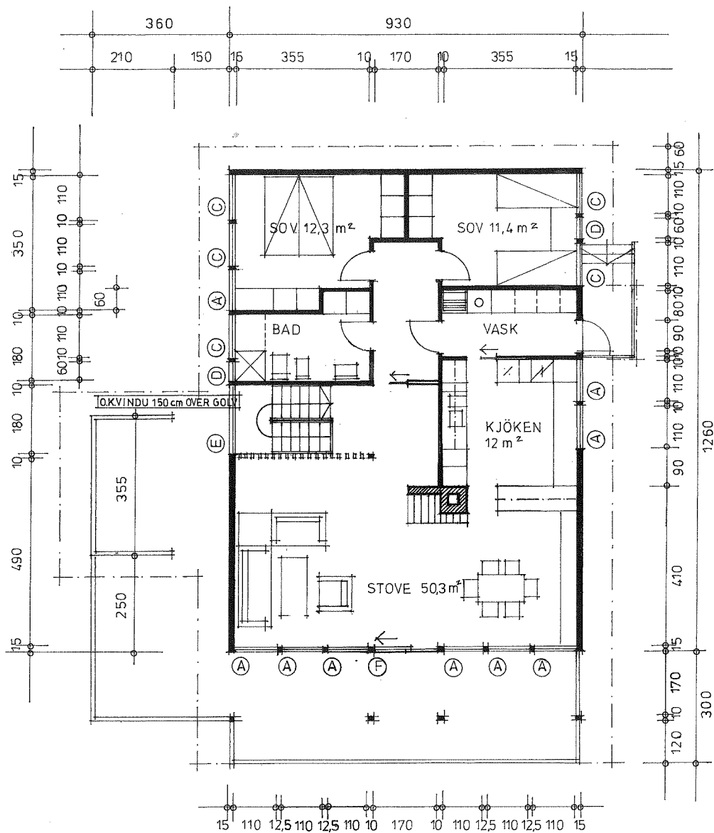
PLAN AV 1. HÖGDA
