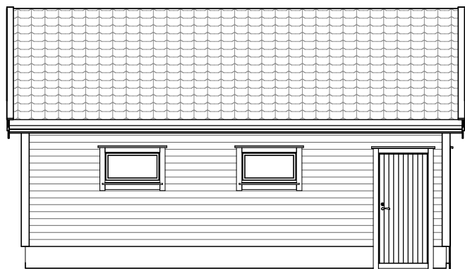
FASADE 1 1 : 100
