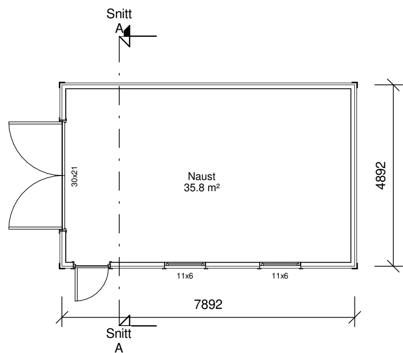
09 ETASJE 1 1 : 100
