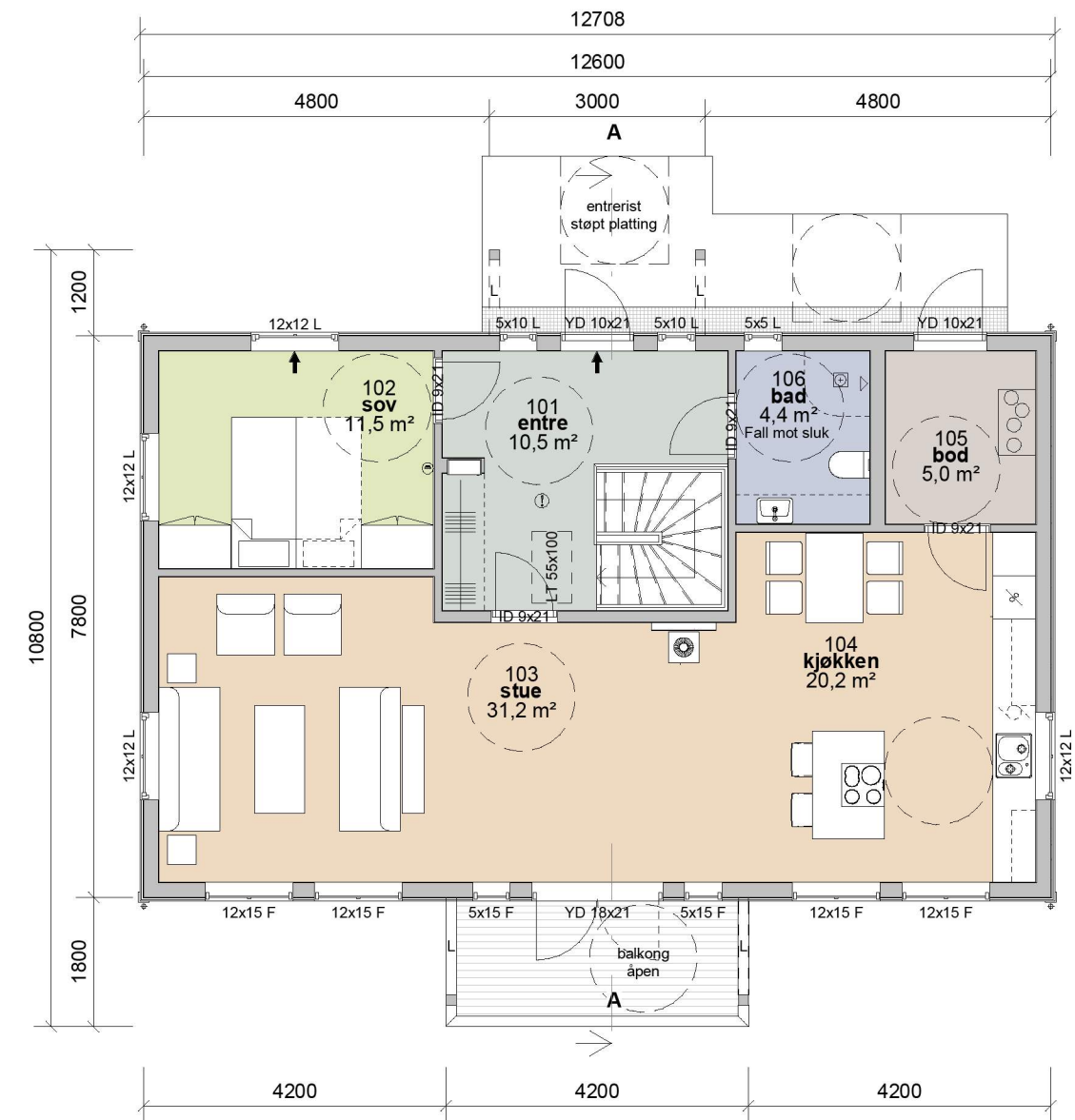
1. Etasje 1 : 100
