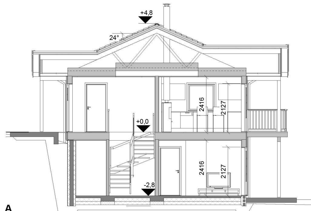
A 1 : 100
