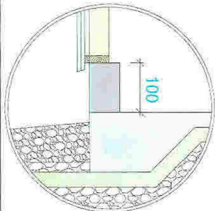
Snitt A
