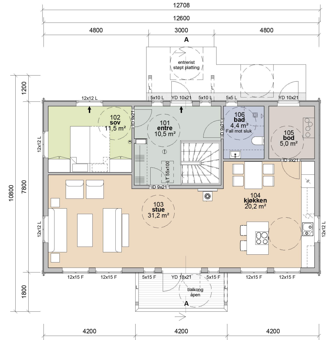
1. Etasje 1 : 100
