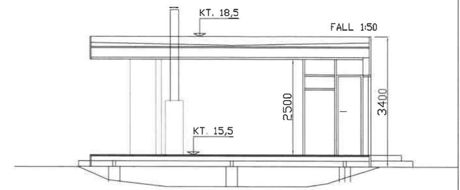
SNITT A-A
