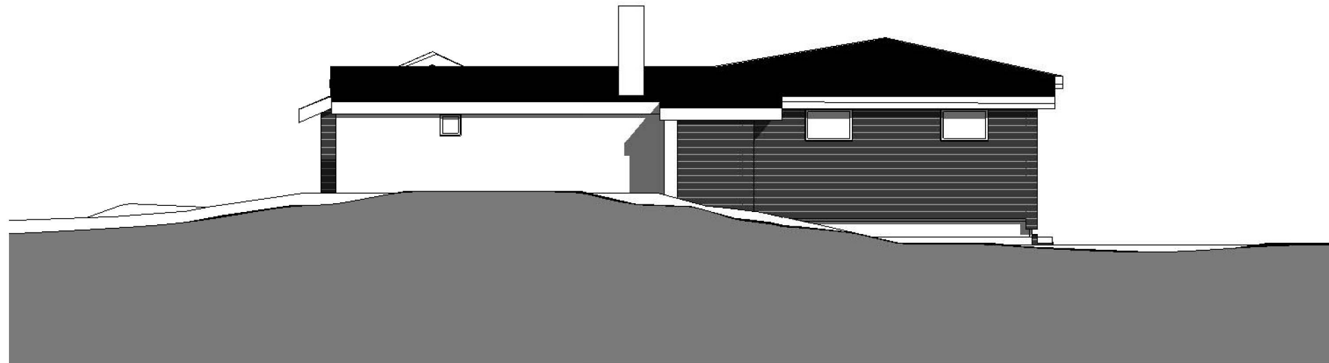
Fasade mot sørvest 1 : 100
