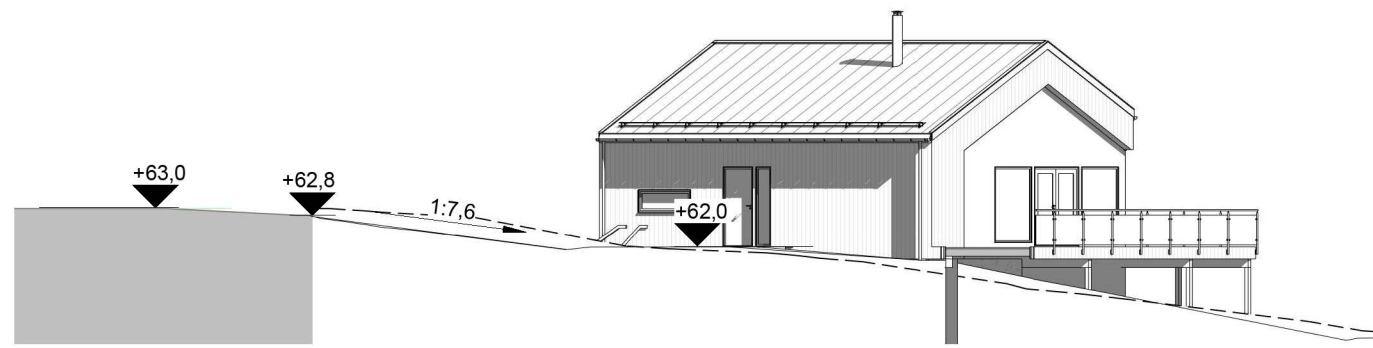
Avkjørsel tomt 1 : 200
