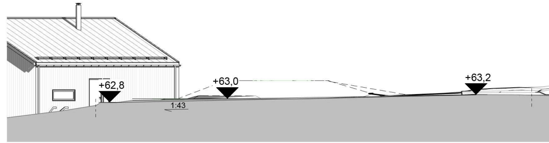
Avkjørsel hovedvei 1 : 200
