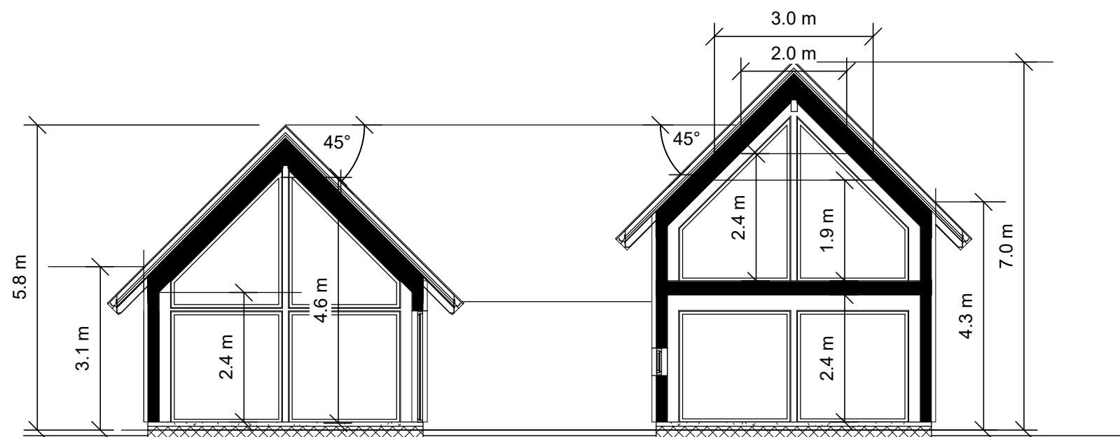
SNITT A-A
