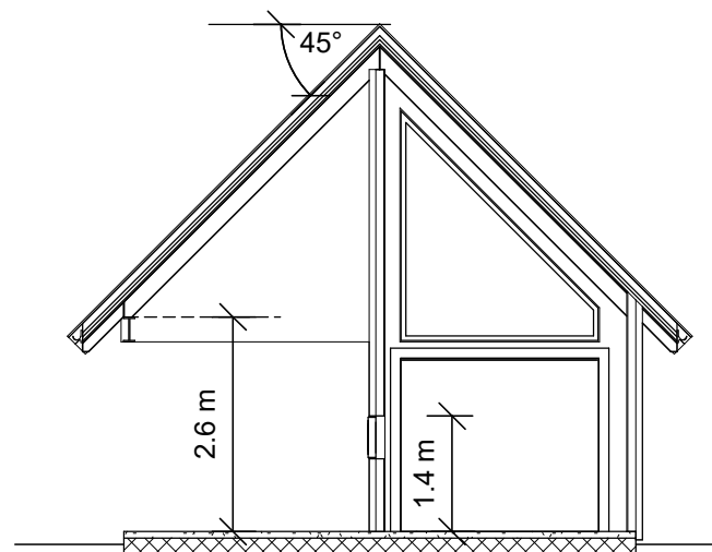
SNITT B-B
