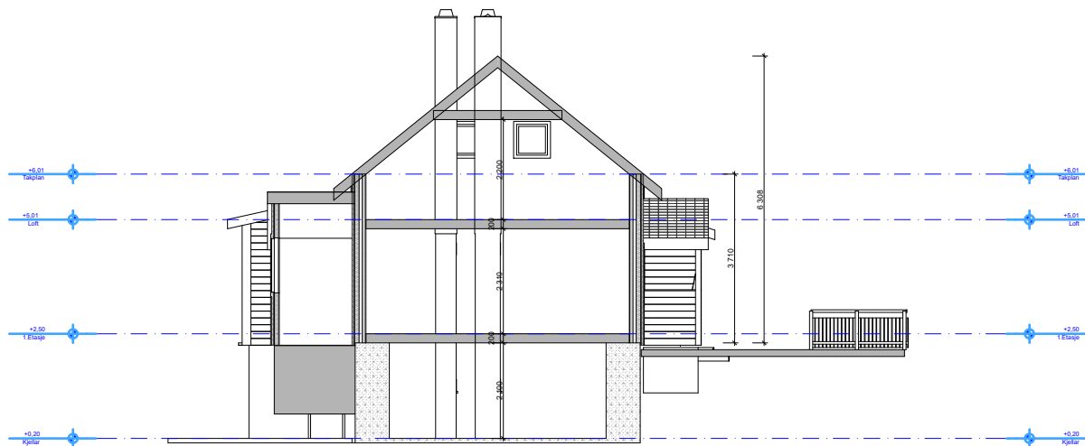
1:150 Snitt A
