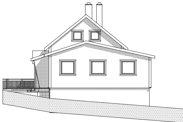
1:200 Fasade Sør
