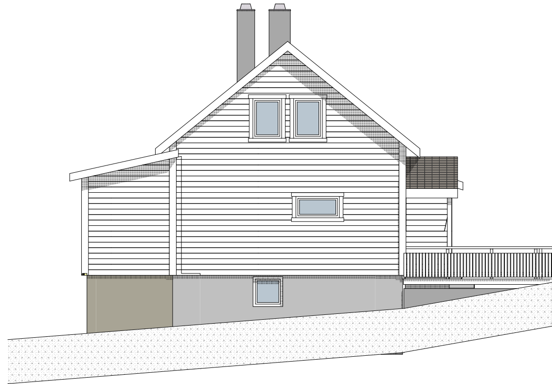
1:100 Fasade Nord
