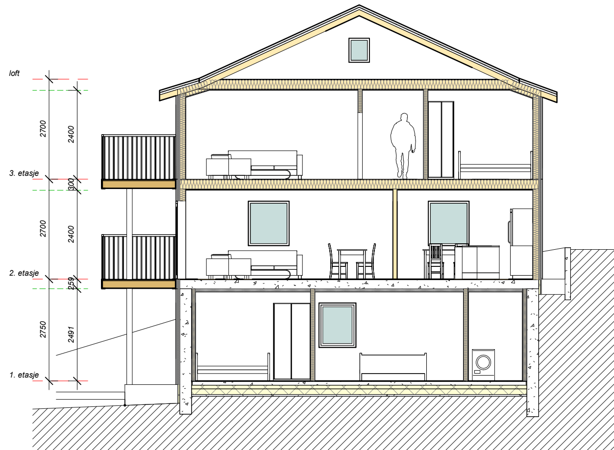
1 Snitt A-A 1 : 100
