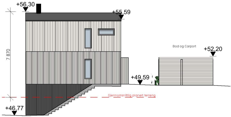
Fasade nordvest
