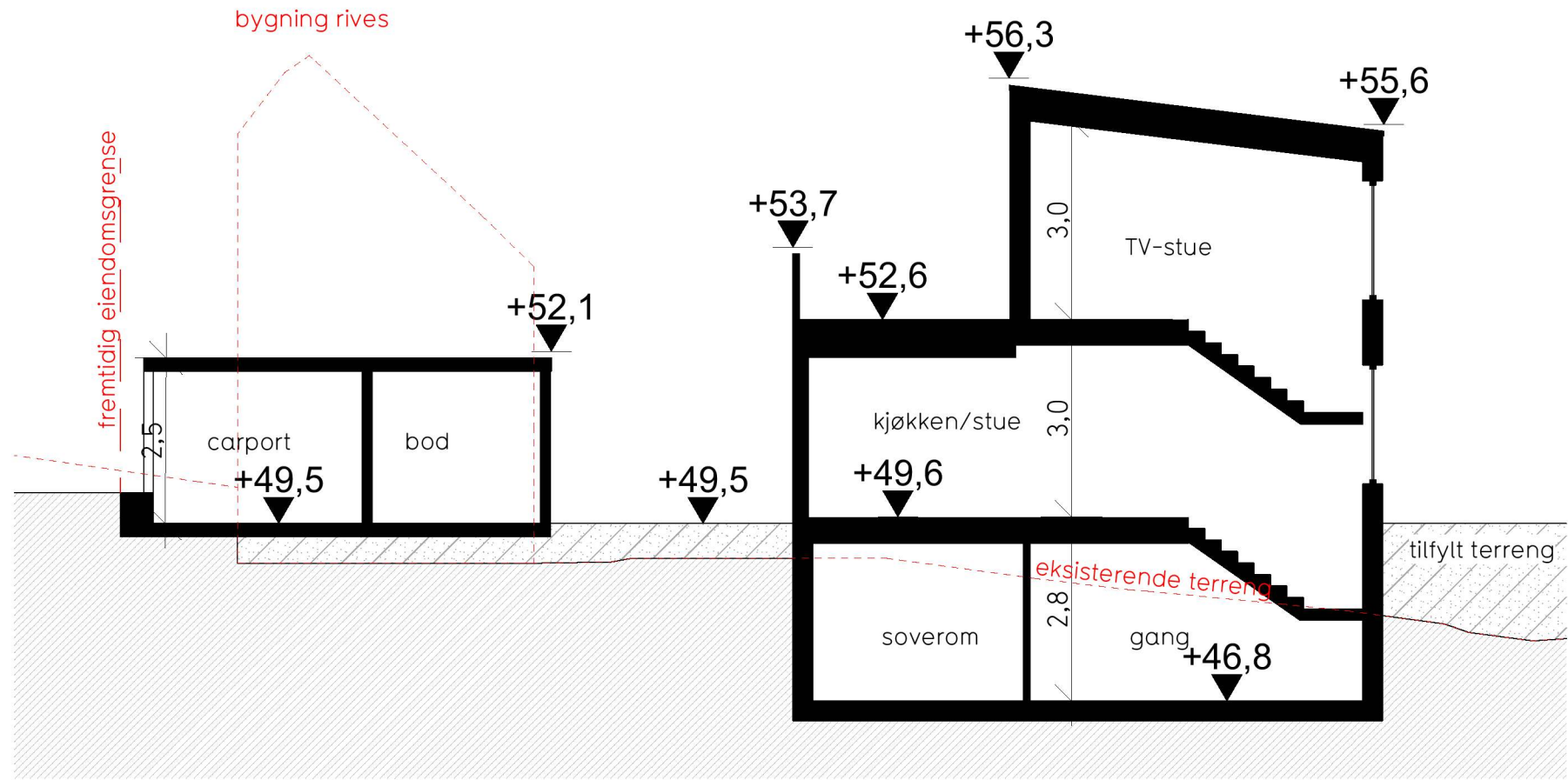
Snitt A Tomt B1b-05
