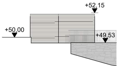
Fasade øst carport 1:200
