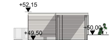
Fasade vest carport:200
