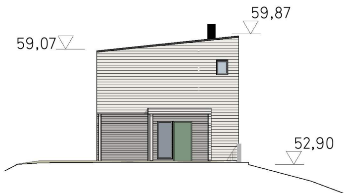
Fasade nordvest 1:200
