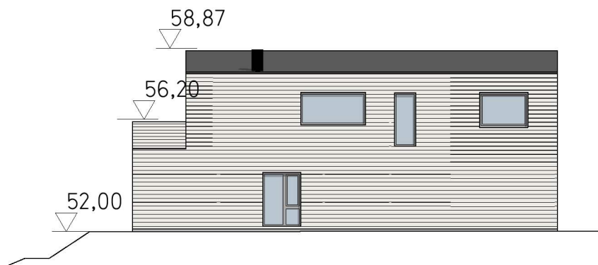
Fasade øst 1:200
