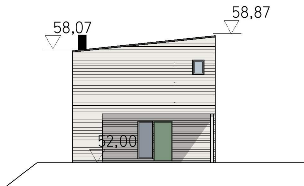
Fasade nord 1:200
