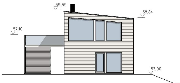
Fasade sør 1:200
