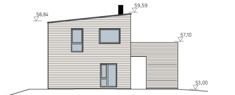
Fasade nord 1:200
