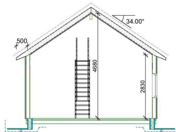
SNITT B-B
