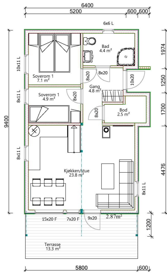
1.ETASJE
