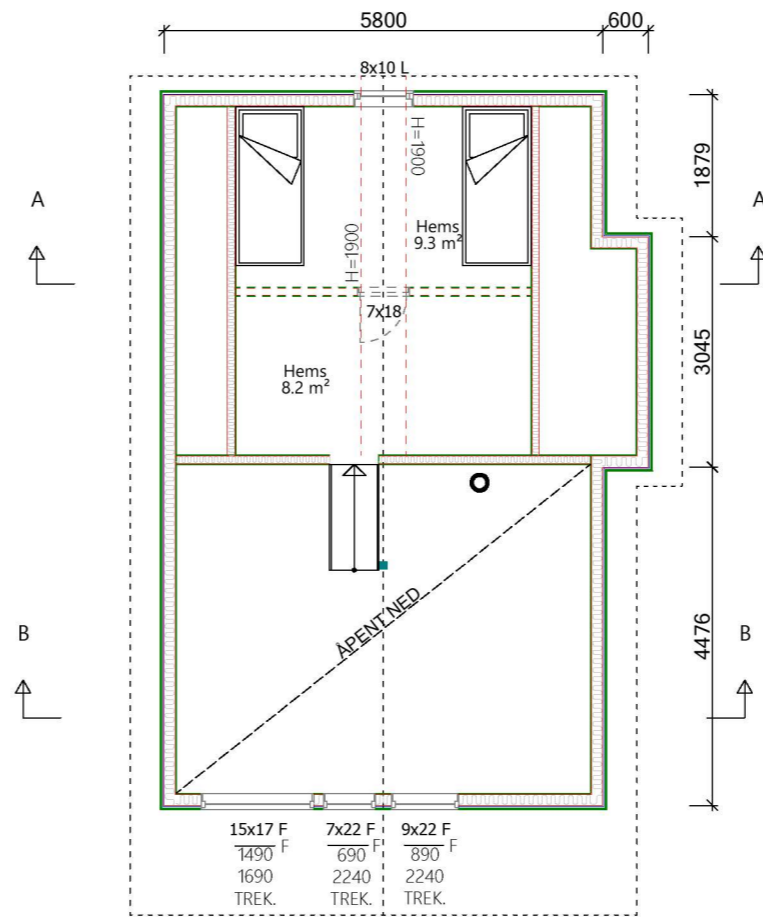
2.ETASJE
