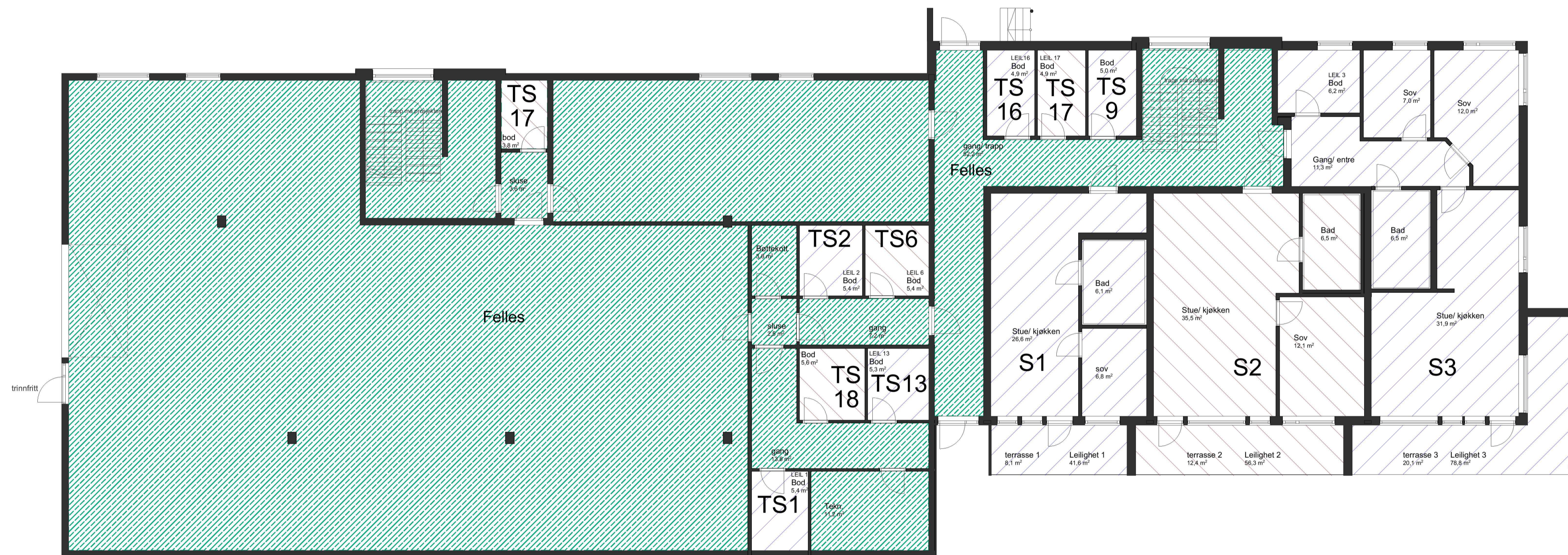
1:100 1. Etasje
