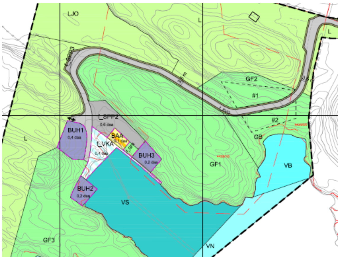
Figur 6-5 Utsnitt av plankartet, for områda som med flest detaljer
