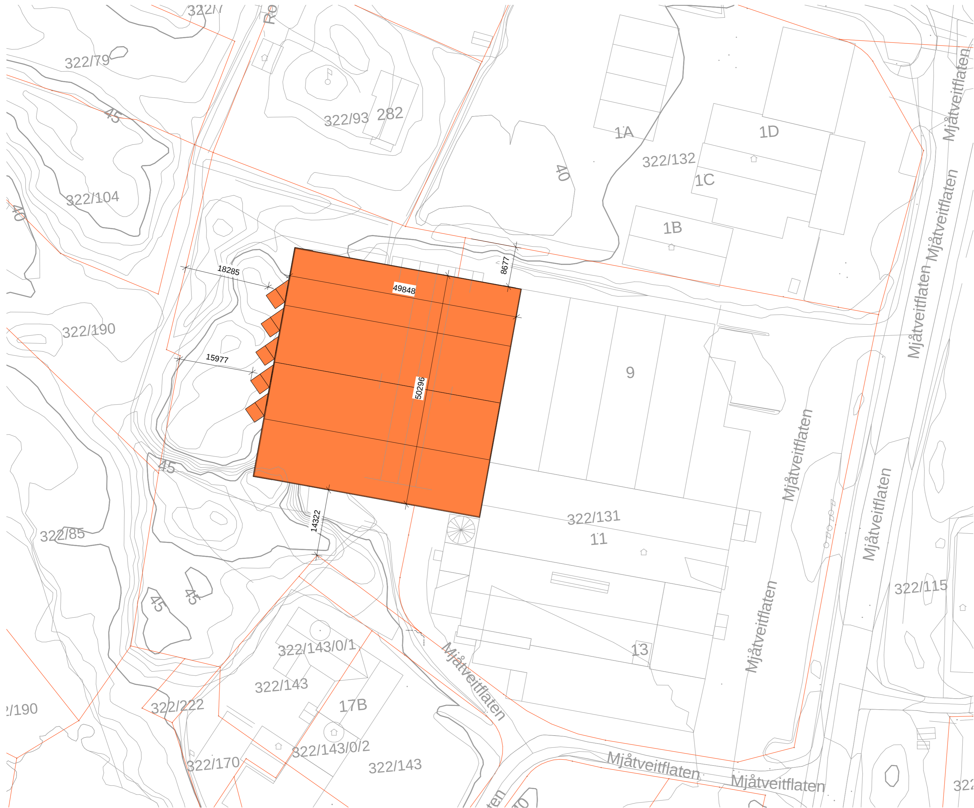
1 Situasjonsplan 1 : 500
