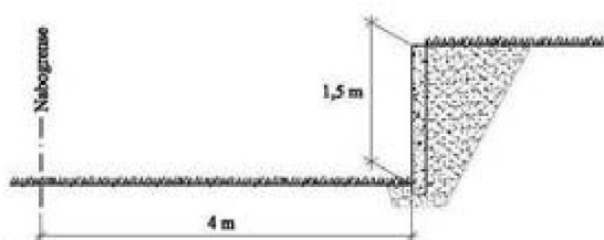
Fig. 2 viser en 1,5 meter høy forstøttemur som må plasseres 4 meter fra nabogrense.
