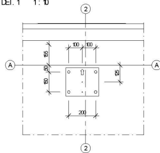
DET. 1 1:10
