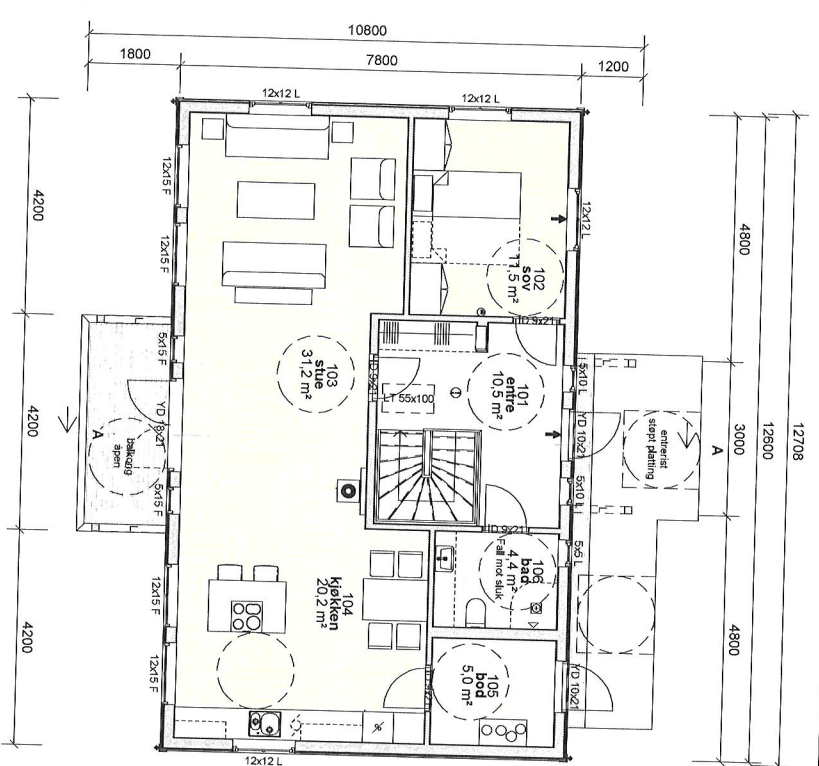
1. Etasje 1 : 100
