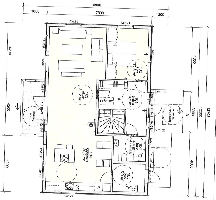
1. Etasje 1 : 100
