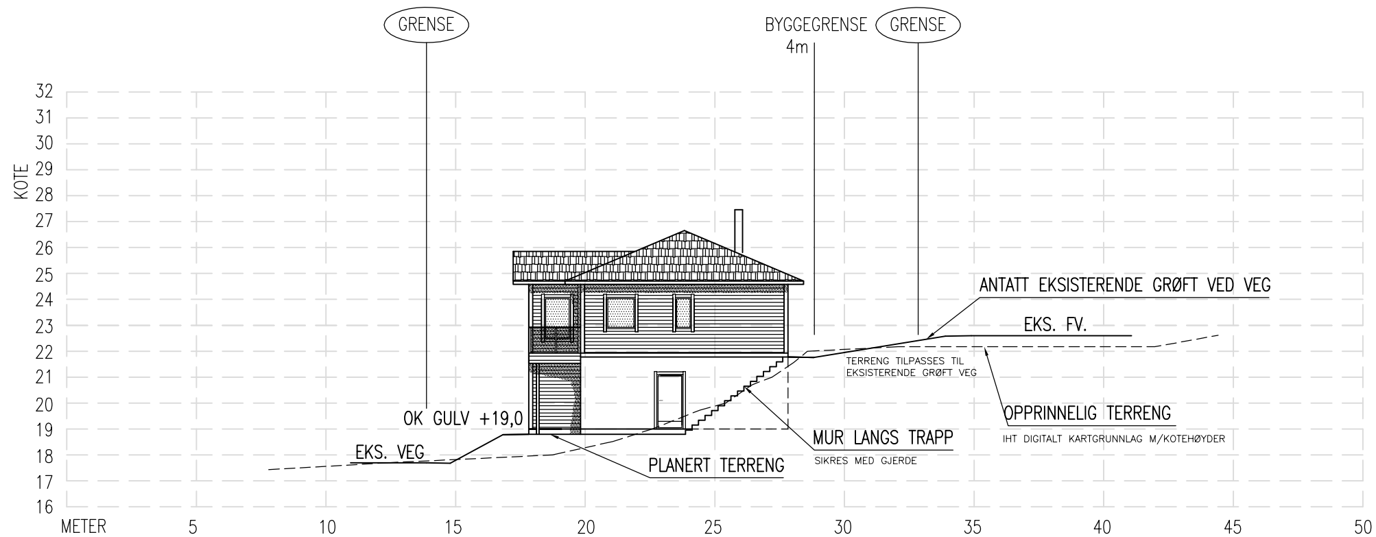
TERRENGPROFIL B-B
