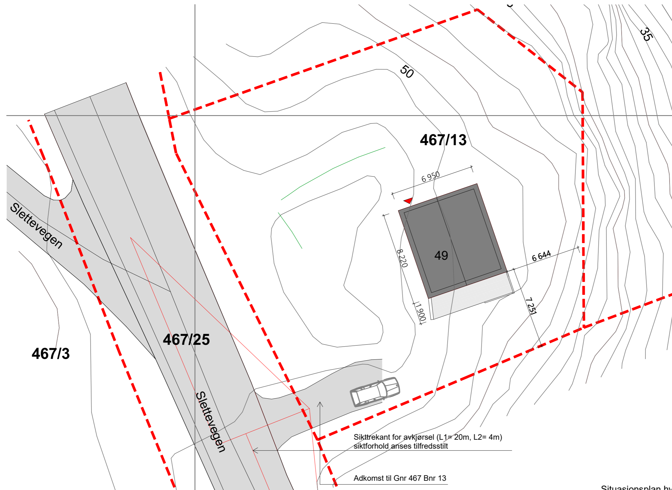
Situasjonsplan hytte, dagens situasjon skala 1:200
