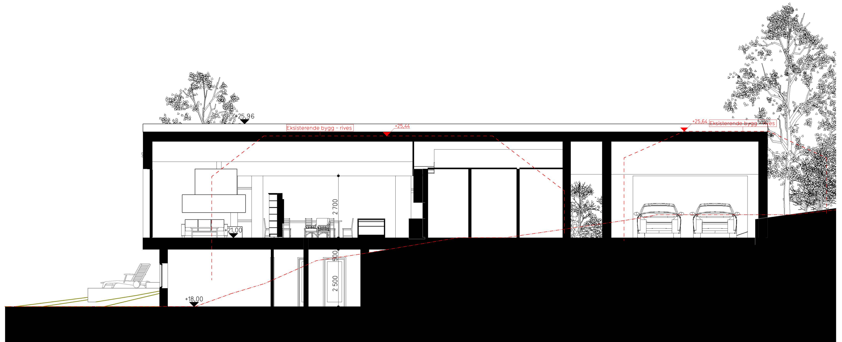
Snitt C
