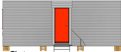
Øst 1 : 100
